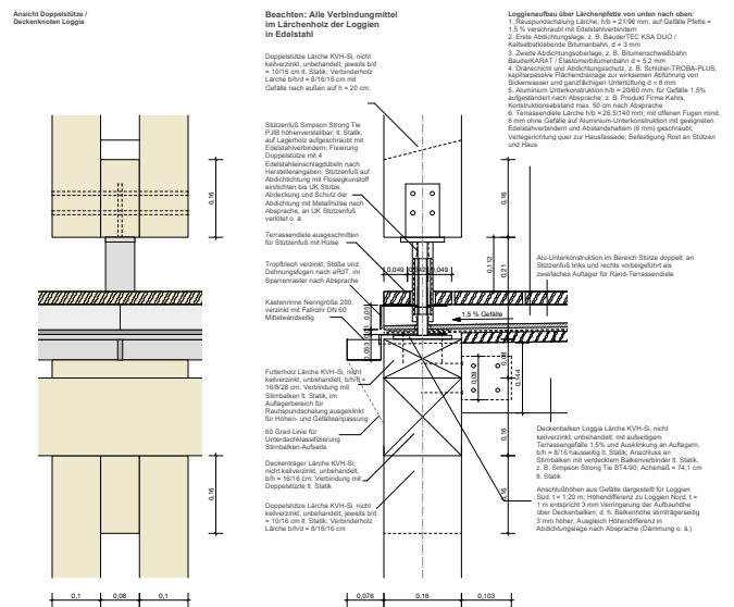
Details Loggia / Planung
